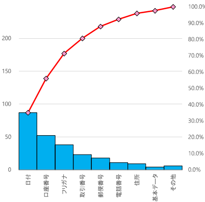
図1 棒グラフの作図
