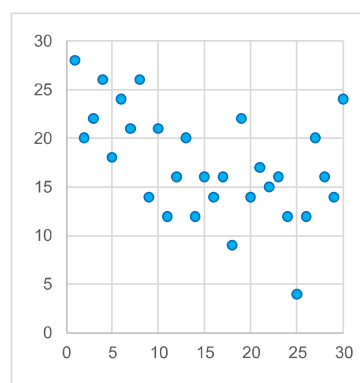
弱い負相関のある場合
