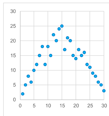
直線的でない関係の場合
