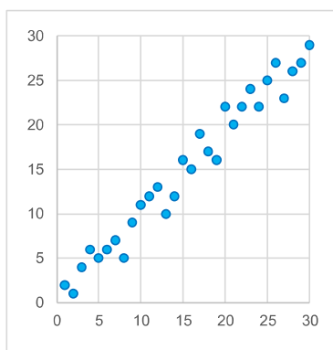
強い正相関のある場合
