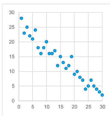
強い負相関のある場合
