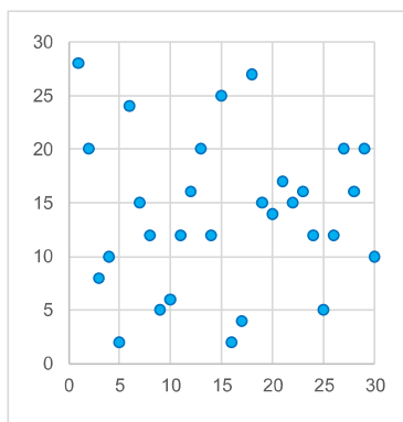
相関のない場合
