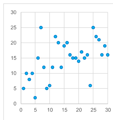
弱い正相関のある場合
